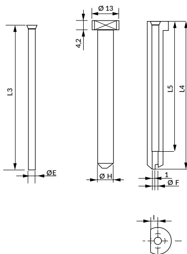
Punzón de embutición / Drawing punch
